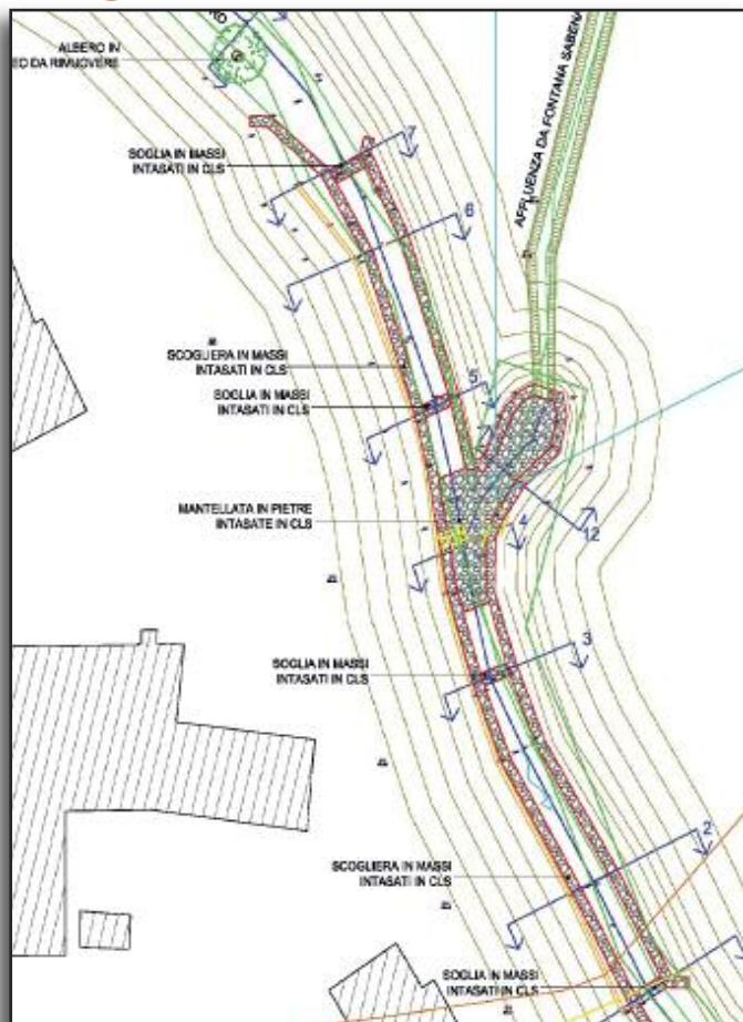
La figura rappresenta la zona centrale dell'intervento di regimazione del rio S. Pietro
