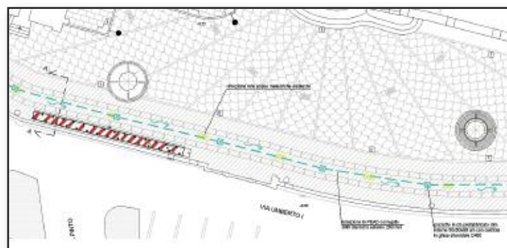
La figura soprastante rappresenta in pianta l'area del consolidamento con evidenziazione in rosso della disposizione dei pali verticali.
